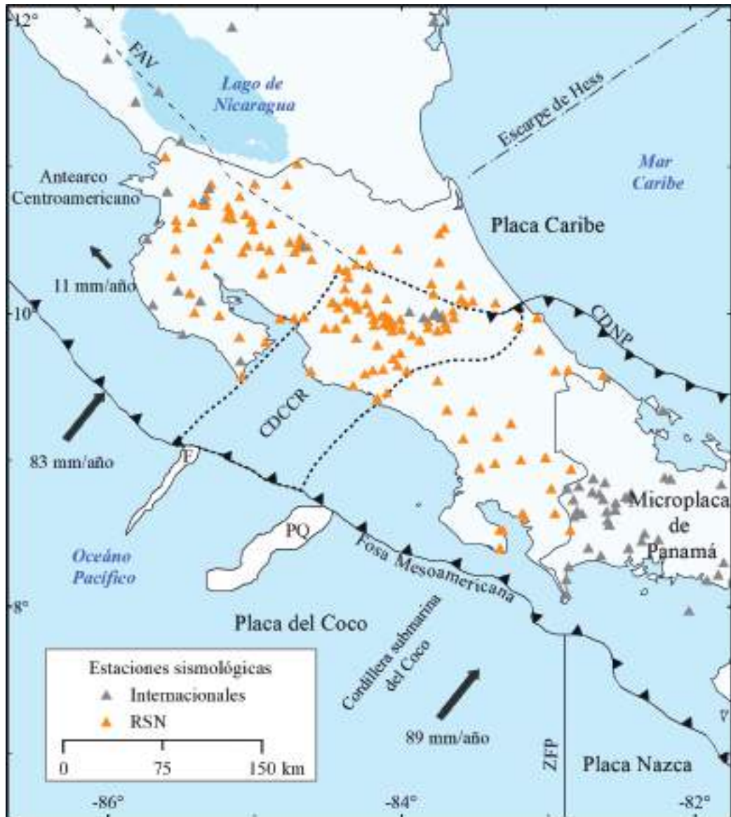
Fig. 1: Contexto tectónico de Costa Rica y estaciones de la Red Sísmica Nacional (RSN: UCR-ICE). La región contenida dentro de la línea gruesa punteada representa el Cinturón Deformado del Centro de Costa Rica (CDCCR). La línea discontinua representa el límite noreste simplificado del Bloque Antearco Centroamericano a lo largo de las Fallas del Arco Volcánico (FAV) de acuerdo con Franco et al. (2012). CDNP es el Cinturón Deformado del Norte de Panamá, F es el monte submarino Fisher, P significa Plateau de Quepos, y ZFP, Zona de Fractura de Panamá.
