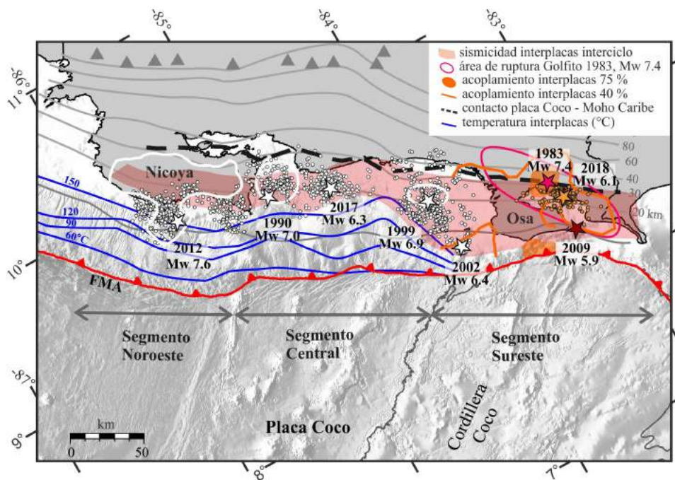
Figura 8. Sísmicidad interplacas interciclo (franja rosada) y ruptura de grandes terremotos en el segmento Pacífico Sureste y comparación con los segmentos Noroeste y Central, en el margen convergente de Costa Rica. La sísmicidad interciclo fue determinada con base en registros de la RSN y otros estudios con redes temporales de tierra y fondo marino (Husen et al. , 2002; DeShon et al. , 2003; DeShon et al. , 2006; Arroyo et al. , 2014a). Se muestra también, para los sismos principales de algunas de las secuencias ocurridas en los últimos 40 años en la zona interplacas, el área de ruptura según: deslizamiento cosísmico para Sámara 2012 (Liu et al. , 2015), imagen tomográfica de un monte submarino subducido para Cóbano 1990 (Husen et al. , 2002), e inversión de ondas de cuerpo para Quepos 1999 (Bilek et al. , 2003) y Golfito 1983 (Tajima y Kikuchi, 1995). Se muestran las réplicas para los sismos de Cóbano 1990 (DeShon et al. , 2003), Quepos 1999 y Osa 2002 (Arroyo et al. , 2014b), Sámara 2012 y Jacó 2017 (Red Sismológica Nacional de Costa Rica, 2017) y Golfito 2018 (este trabajo). Los contornos del techo de la placa del Coco fueron estimados por Lücke y Arroyo (2015), las temperaturas en la zona interplacas por Ranero et al. (2008), y el acoplamiento interplacas en el sureste de Costa Rica por Kobayashi et al. (2014). Los triángulos grises representan los volcanes activos. La cordillera del Coco se delinea según el contorno batimétrico de 2000 m de profundidad. FMA significa Fosa Mesoamericana.
