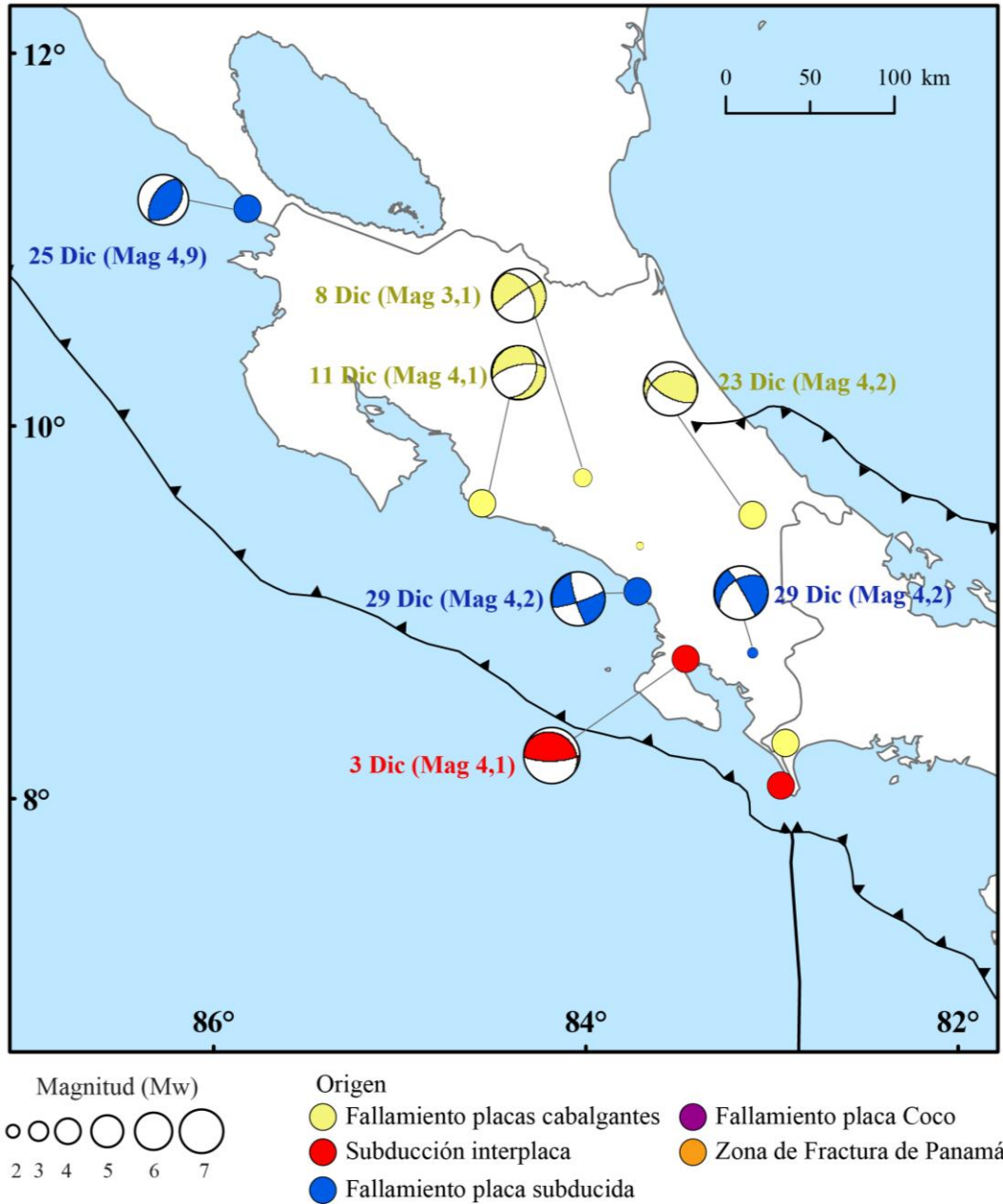
Figura 5: Origen de los sismos sentidos en Costa Rica durante diciembre del 2024, Se muestra el mecanismo focal y la fecha y Mw entre paréntesis para algunos sismos del mes. El color de los epicentros y mecanismos focales indica el origen de acuerdo con la simbología en la base de la figura.
