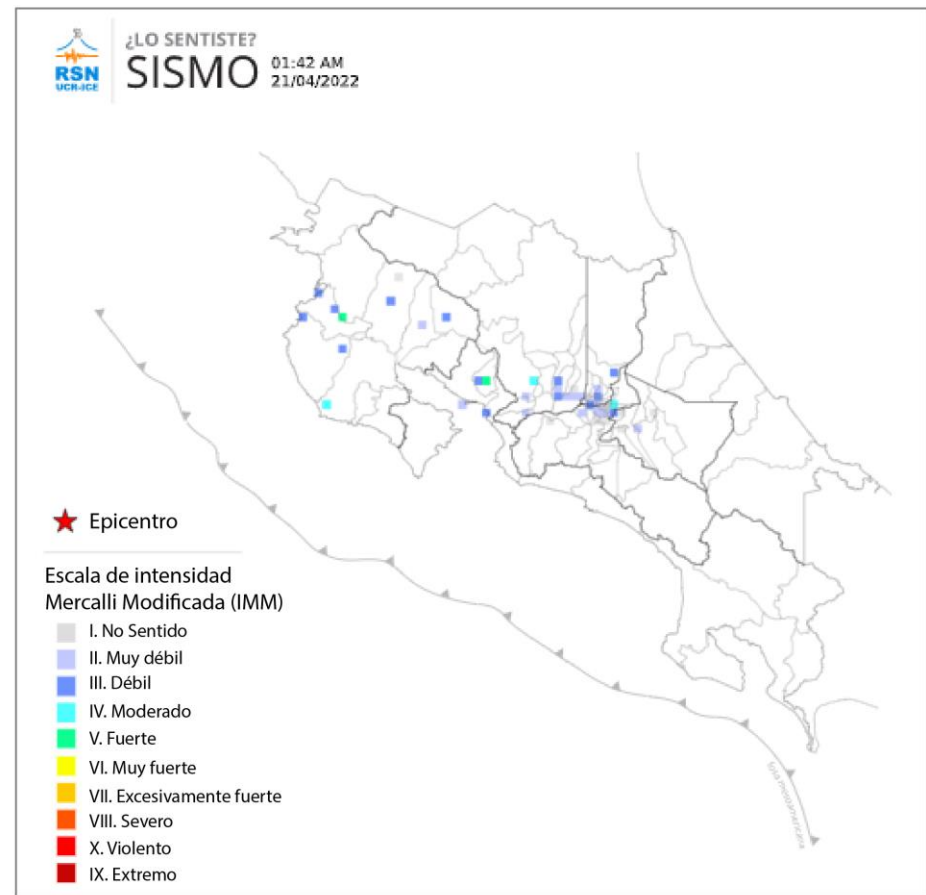
Figura 7: Intensidades reportadas por usuarios a través del módulo ‘¿Lo Sentiste?’, de la aplicación RSN para el evento del día 21 a la 1:42 a. m. (Mw 6,5), ocurrido a 23 km de profundidad, 109 km al suroeste de Managua, Nicaragua.
