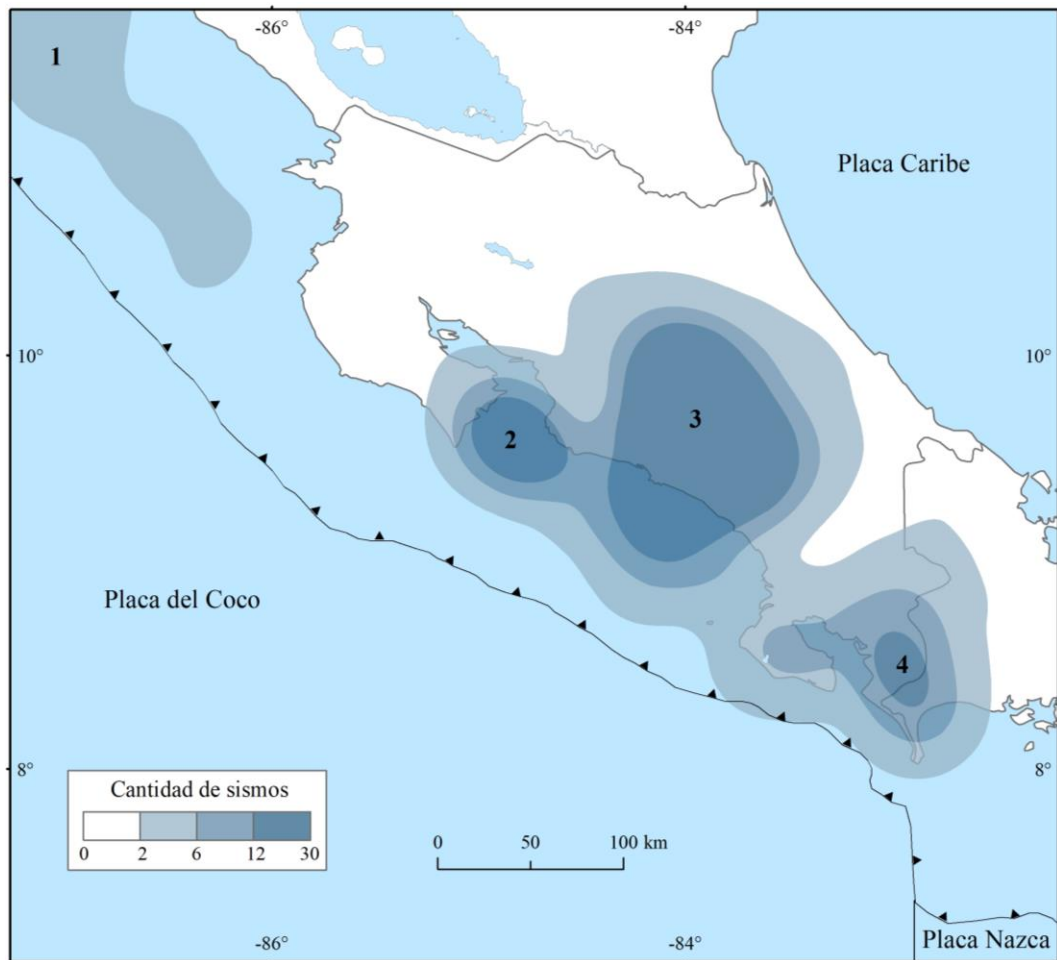
Figura 3: Distribución espacial de la cantidad de sismos durante abril del 2022. Los cúmulos 1, 2, 3 y 4 corresponden con las zonas con la mayor cantidad de sismos localizados.
