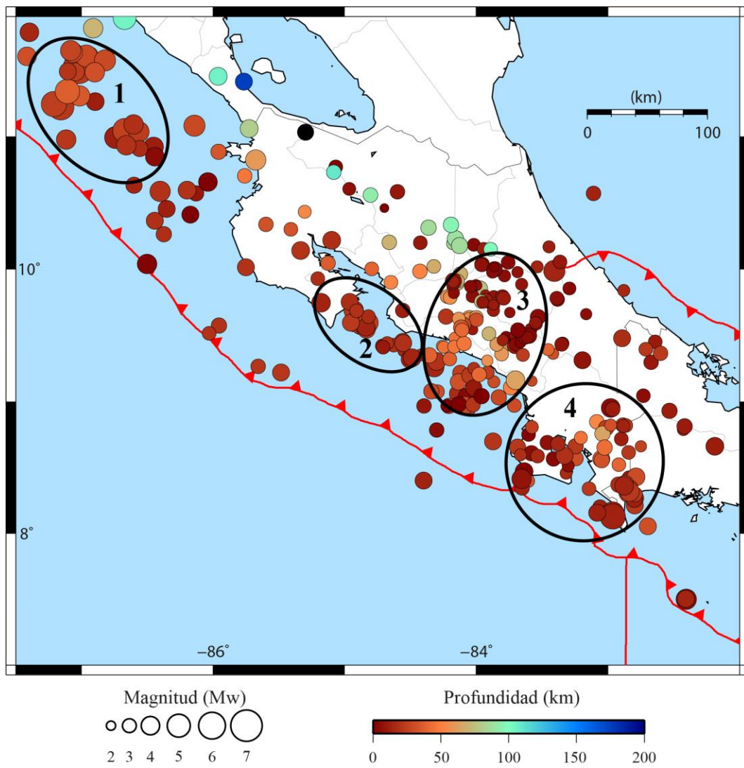
Figura 2: Sismos localizados por la RSN en el territorio nacional durante abril del 2022. Los cúmulos 1, 2, 3 y 4 corresponden a las zonas con la mayor cantidad de sismos localizados.
