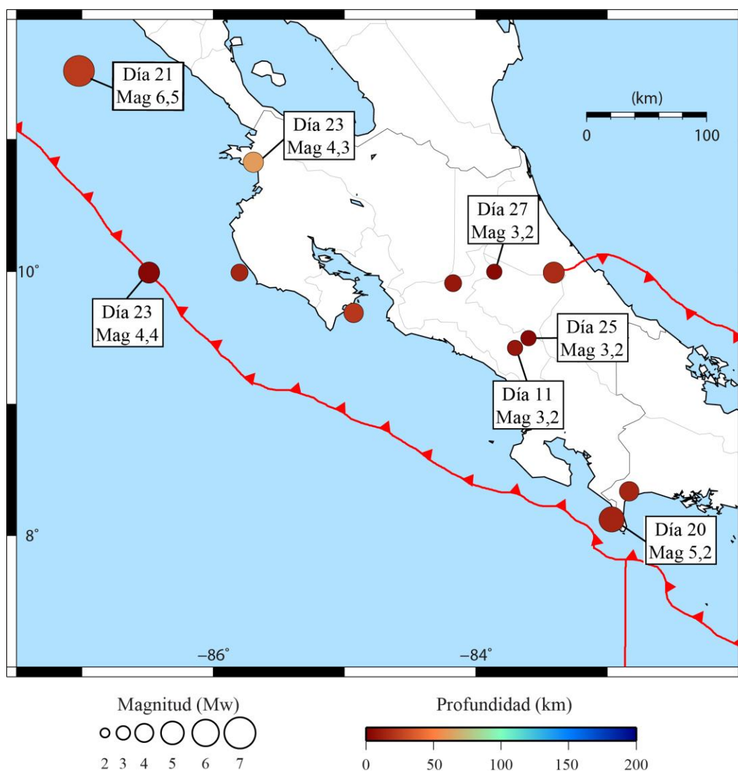
Figura 5: Sismos sentidos en Costa Rica ocurridos durante abril del 2022, originados en el territorio nacional y alrededores. Se indica la magnitud M_w para algunos sismos mencionados en este boletín.
