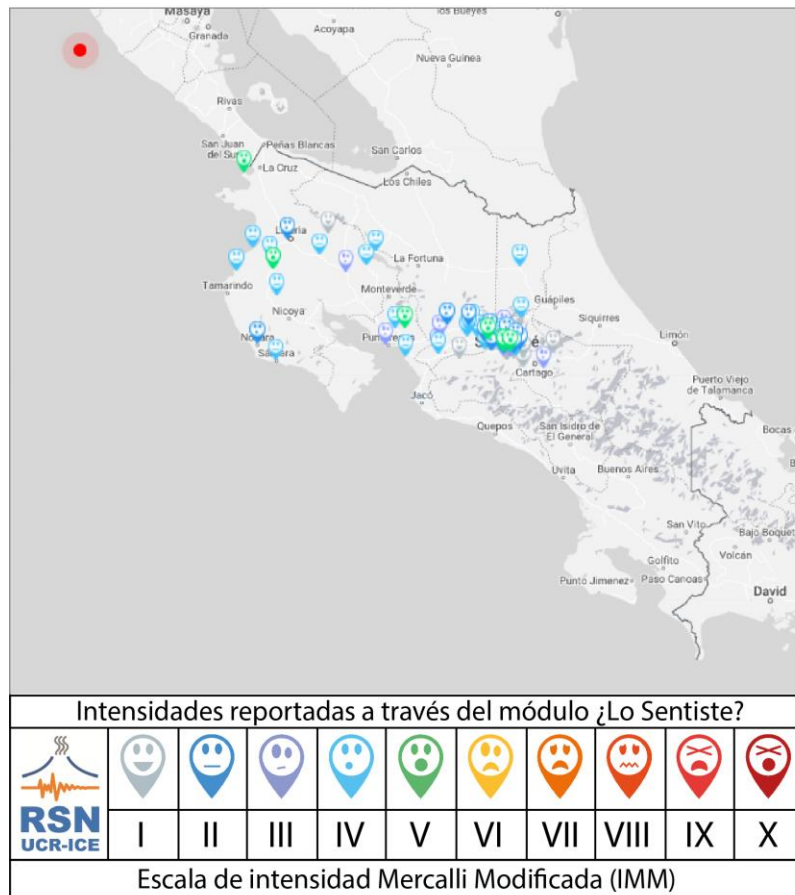
Figura 7: Intensidades reportadas por usuarios a través del módulo ‘¿Lo Sentiste?’, de la aplicación RSN para el evento del día 21 a la 1:42 a. m. (Mw 6,5), ocurrido a 23 km de profundidad, 109 km al suroeste de Managua, Nicaragua.
