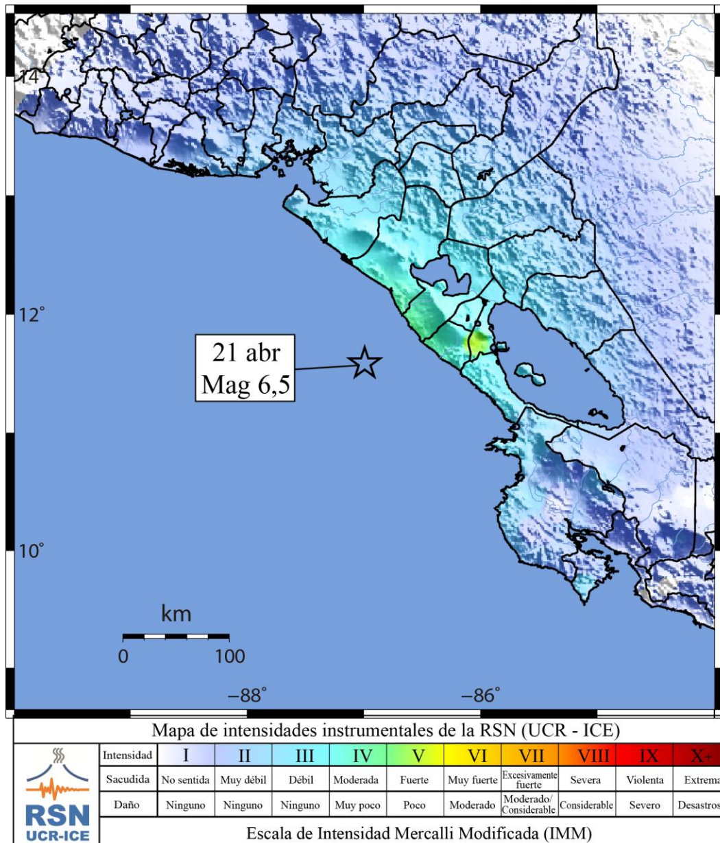
Figura 6: Intensidades máximas registradas por la red de instrumentos de la RSN durante abril del 2022, debido al sismo del día 21 a la 1:42 a. m. (Mw 6,5), ocurrido a 23 km de profundidad, 109 km al suroeste de Managua, Nicaragua.
