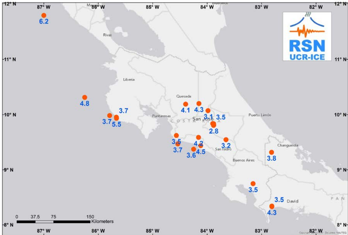
Mapa de los sismos sentidos durante el mes de junio del 2013 (RSN)
