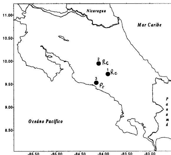
Figura1. Sismos sentidos, octubre 1997. Los eventos se muestran con círculos rellenos y se enumeran en orden de ocurrencia de acuerdo al cuadro 1.
