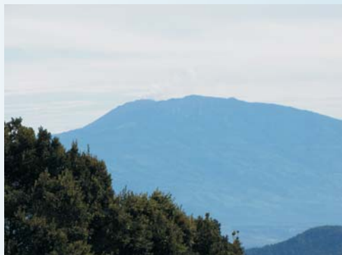
Penacho de gases del volcán Turrialba, desde La Georgina (Interamericana Sur), 28 de mayo del 2010, foto cortesía de Raúl Mora.
